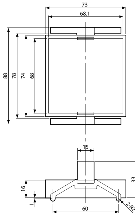
计数器挡块
