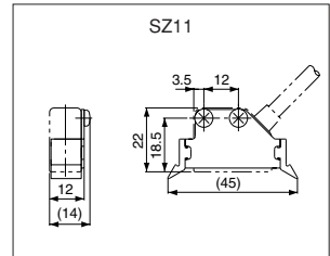
外形寸法
